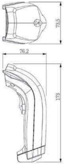
外形尺寸圖
